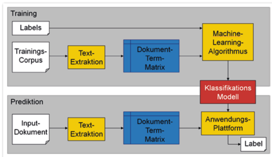
Abbildung 2: Training und Anwendung eines Klassifikationsmodells durch überwachtes Lernen
