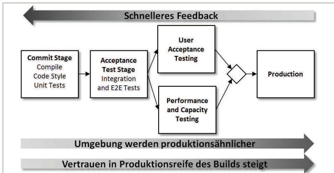
Abbildung: Build Pipeline Stages
